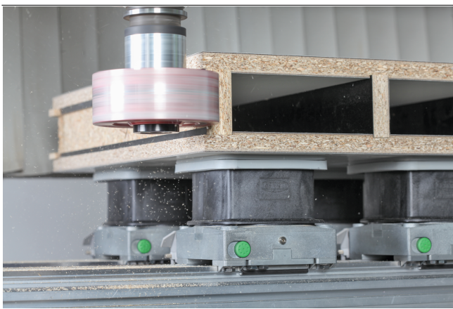
Bloc de bridage par le vide VCBL-B pour le bridage de panneaux d'aggloméré
