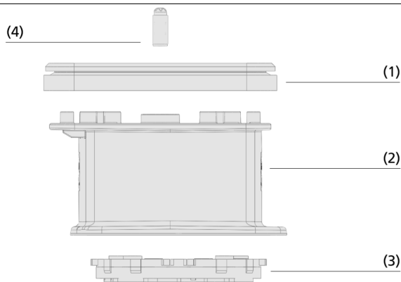
Composition des Blocs de bridage VCBL-B
